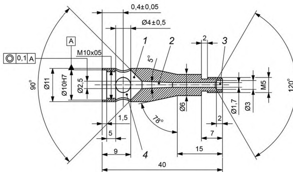
Рисунок Г.8 — Стабилизатор пламени горелки
