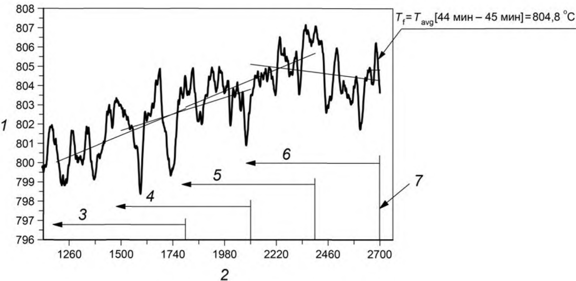
1 — температура, °С; 2 — время, с; 3 — смещение [20 мин — 30 мин] = 2,76 °С; 4 — смещение [25 мин — 35 мин] = 2,15 °С; 5 — смещение [30 мин — 40 мин] = 2,80 °С; 6 — смещение [35 мин — 45 мин] = 0,84 °С; 7 — время окончания испытания, равное 45 мин.
