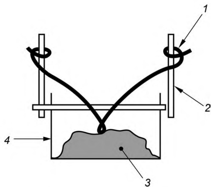
Рисунок Д.2 — Метод «тигля»
